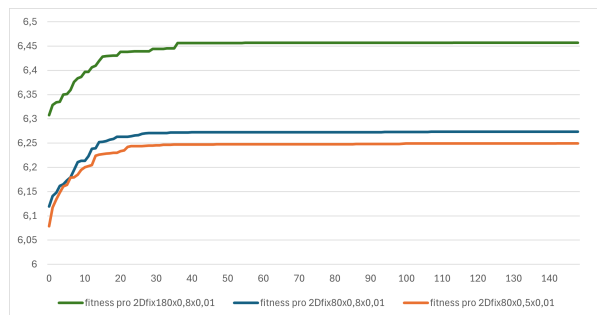
Obr. 7: Porovnání rychlosti konvergence a kvality řešení pro GA P_m = 0,01 .
