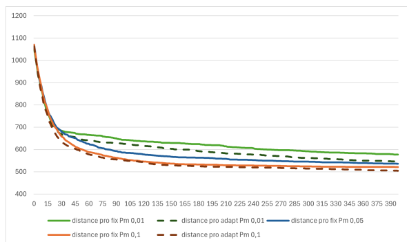
Obr. 9: Porovnání rychlosti konvergence a kvality řešení pro GA různé P_m .
