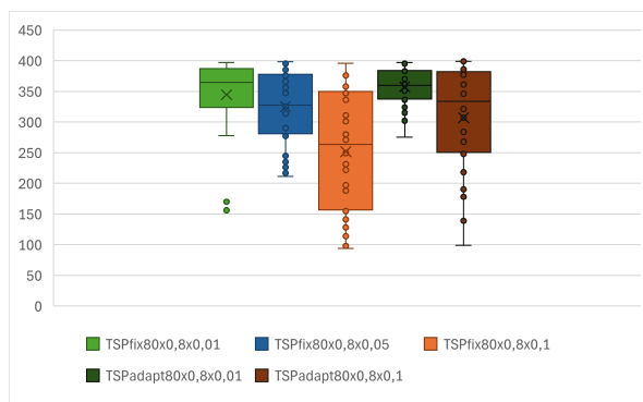
Obr. 10: Porovnání variance best_gen pro GA TSPfix80x0,8xPm a TSPadapt80x0,8xPm.
